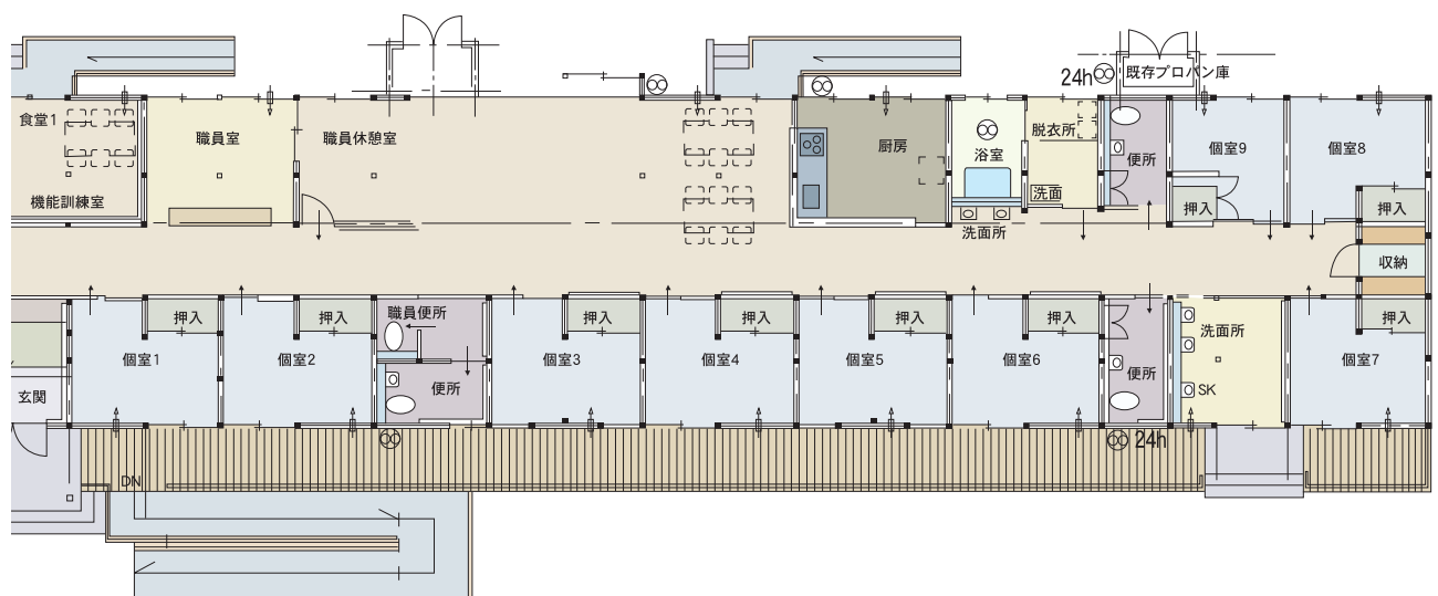
グループホーム のんびり館「施設図」
